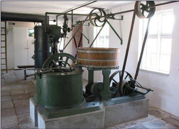
Figur 18. Den sorte dampmaskine i baggrunden. vi Fra Hjedding Museumsmejeri.
